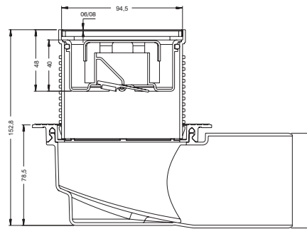
Ø 70 SIDE Outlet
