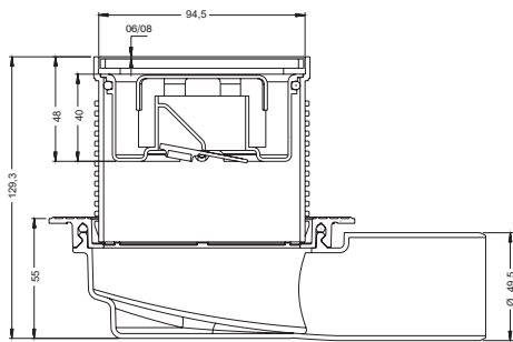
Ø 50 SIDE Outlet
