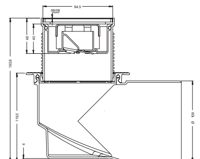
Ø 100 SIDE Outlet
