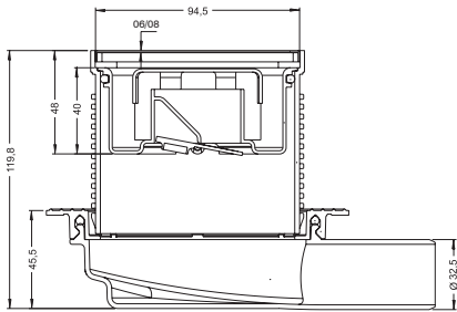
Ø 32 SIDE Outlet
