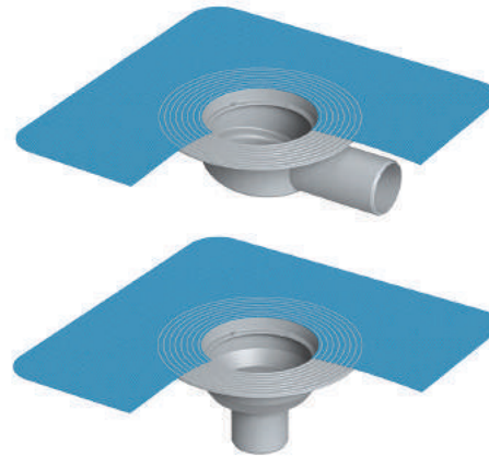
Siphon lower body / пластичное тело الجسم السفلي
